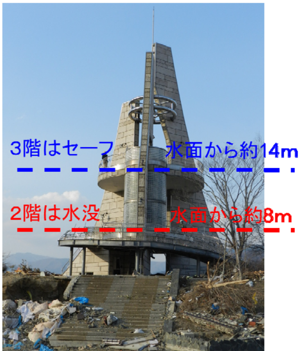
写真4 港湾埋立地内にある避難タワー（大船渡市サンアンドレス公園）
