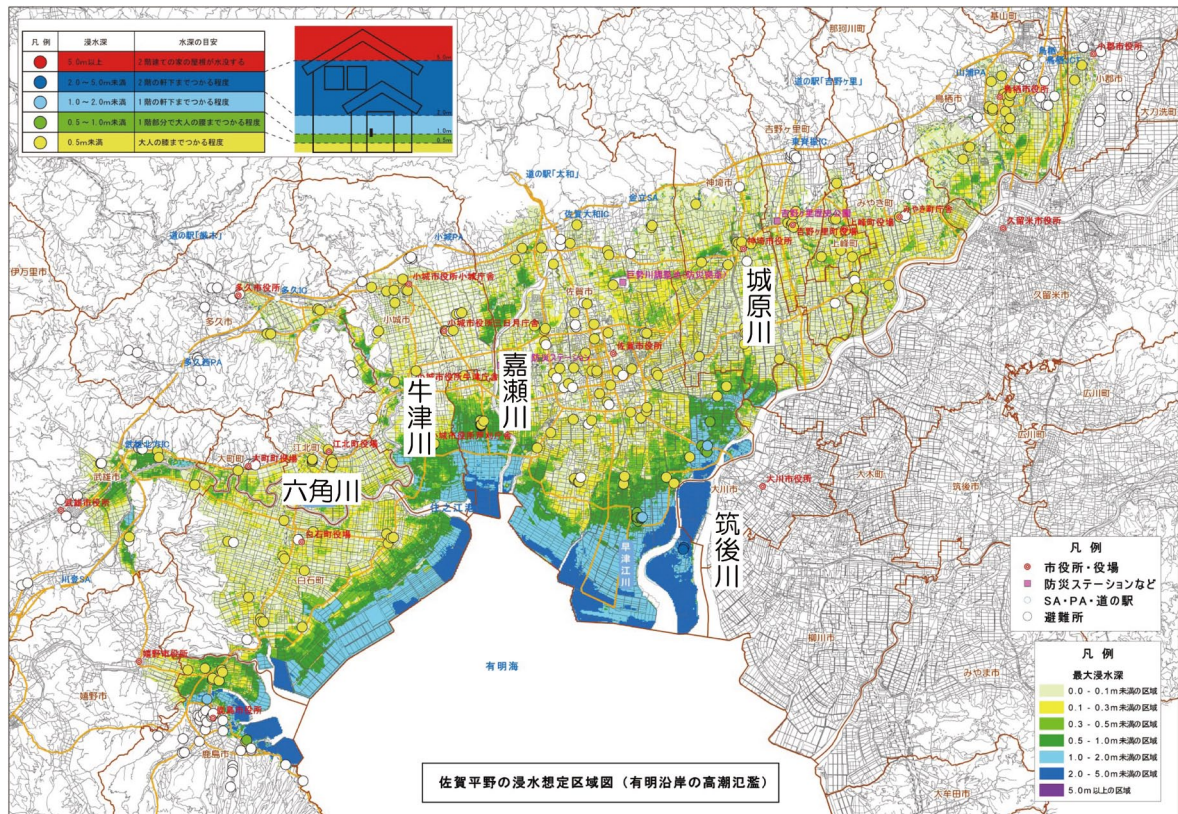
口絵写真－2 佐賀平野における台風時の降雨・高潮がもたらす浸水の想定区域 2)
