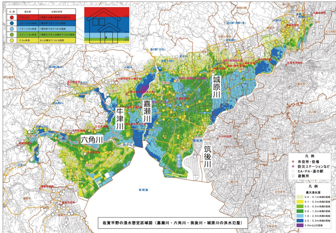
口絵写真－1 佐賀平野の浸水想定区域（筑後川・城原川・嘉瀬川・六角川の洪水氾濫） 2)
