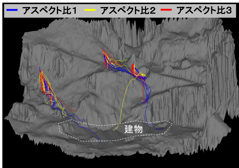
口絵写真-2 落石経路（アスペクト比で色分け）
