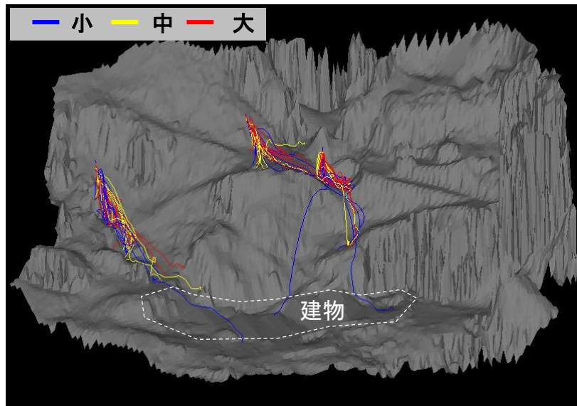
口絵写真-1 落石経路（サイズで色分け）
