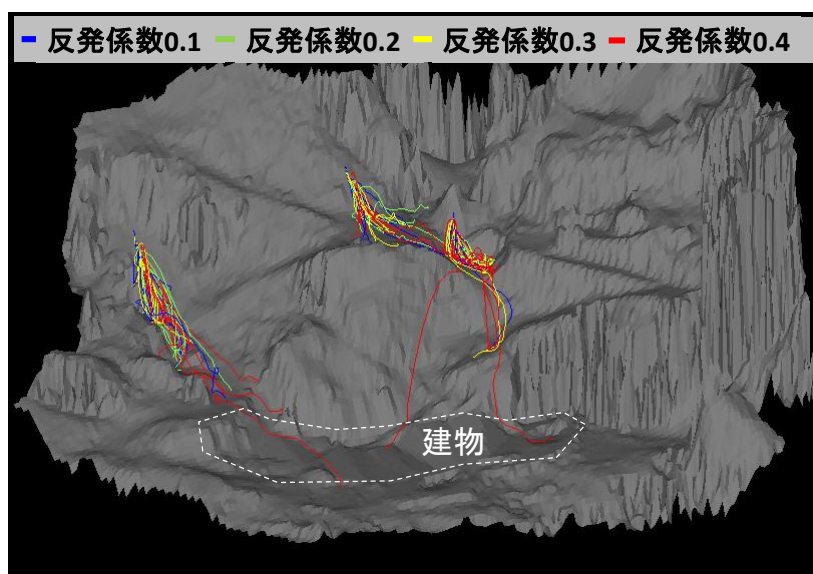
口絵写真-3 落石経路（反発係数で色分け）
