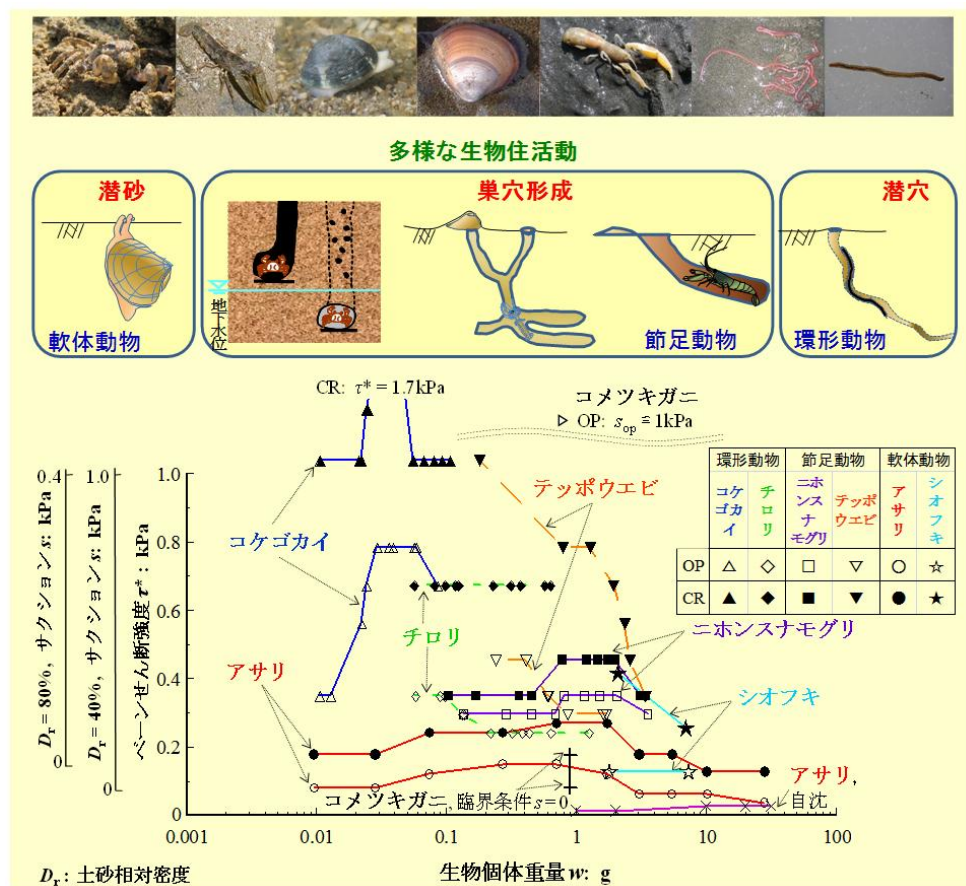
口絵写真－57 多種多様な生物住環境診断チャート (OP：適合土砂環境場、CR：限界土砂環境場を表す)
