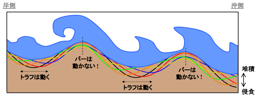
口絵写真－56 潮間帯砂州の動的安定原理の解明に基づくバリア地形の概念図 －東京湾葛西沖の浅場造成事業の設計に活用－
