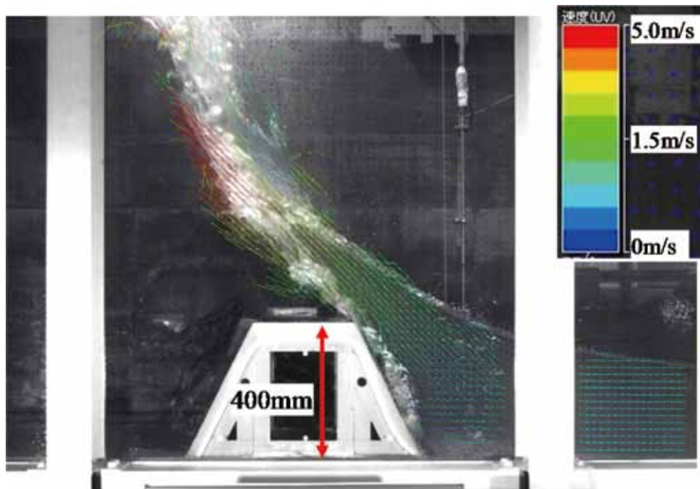
口絵写真－1 画像解析による流速分布測定結果例
