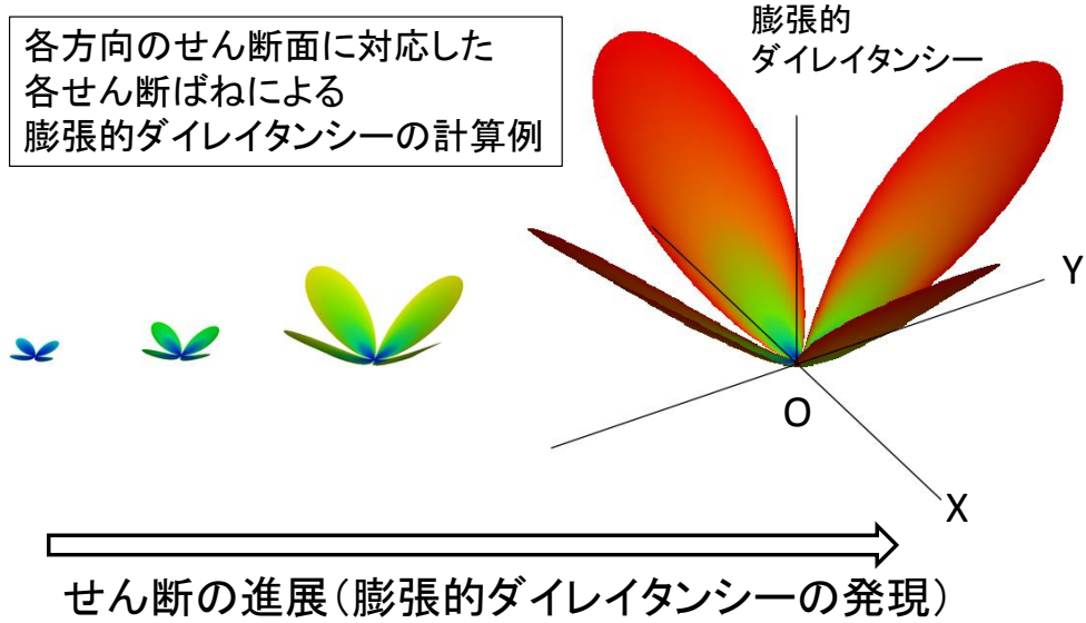
口絵写真-1 カクテルグラスモデルにおける誘導異方性
