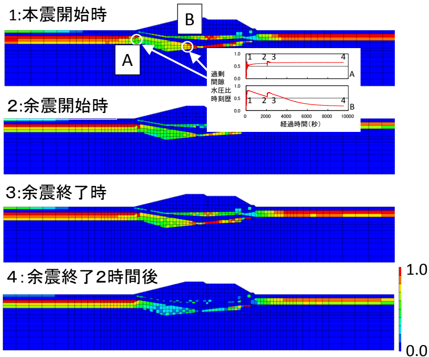
口絵写真-2 2011年東日本大震災時の利根川河川堤防の再現解析
