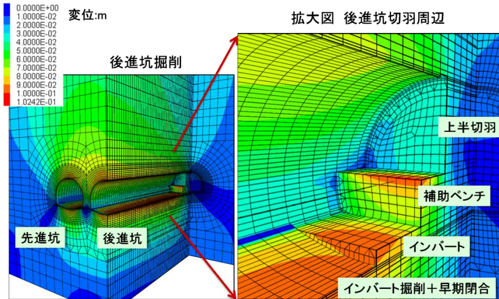
口絵写真-11 後続トンネル掘削過程時のモデルと変位分布
