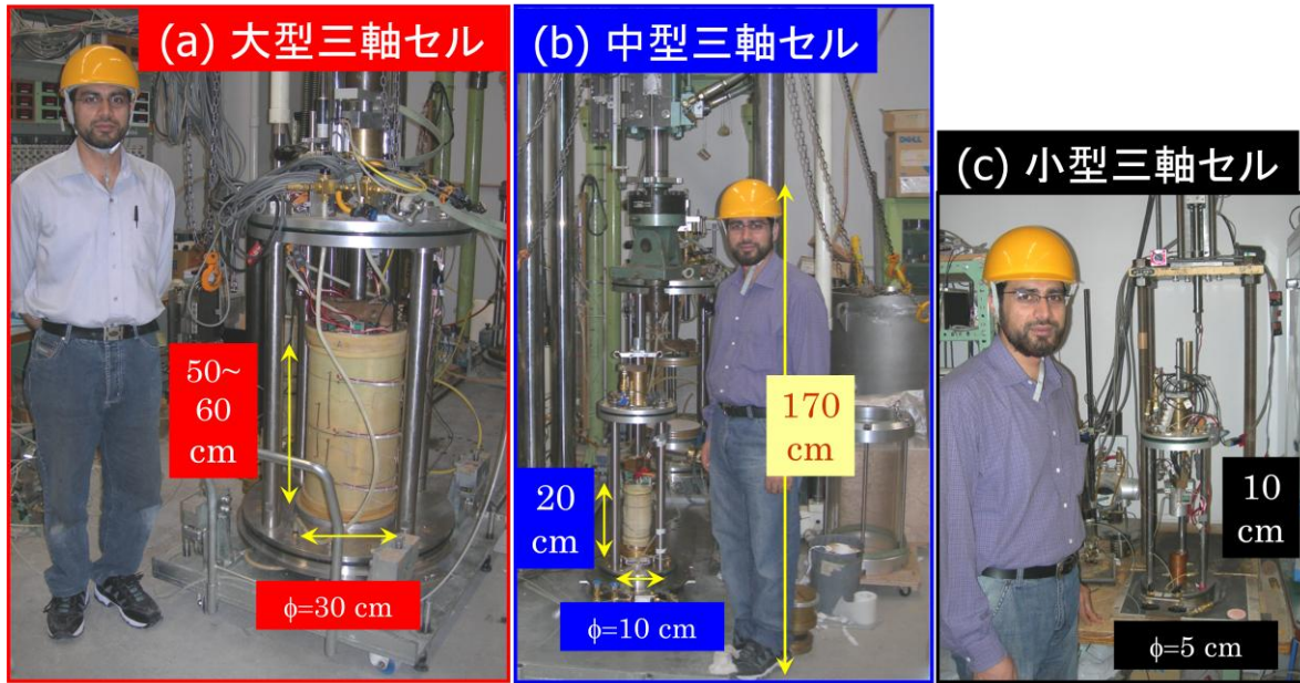
口絵写真-2 大型・中型・小型三軸圧縮試験の供試体と三軸セル
