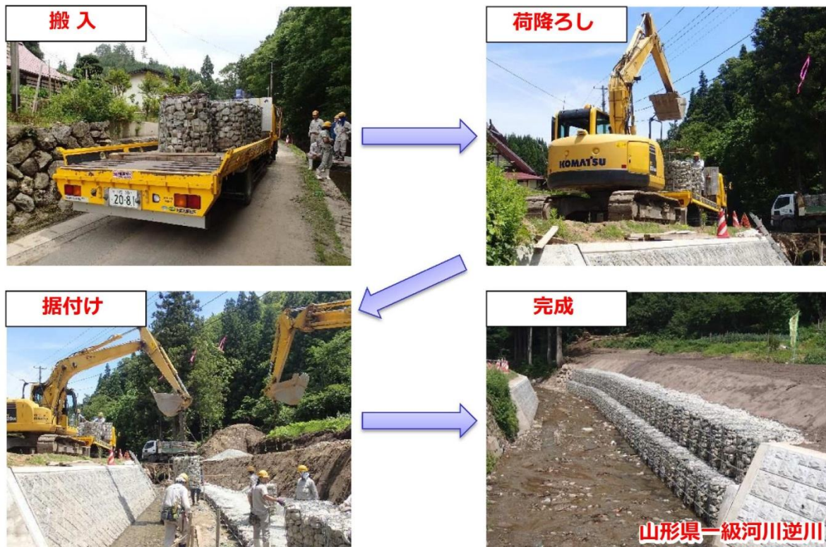
口絵写真-1 「かご丸くん」 施工事例
