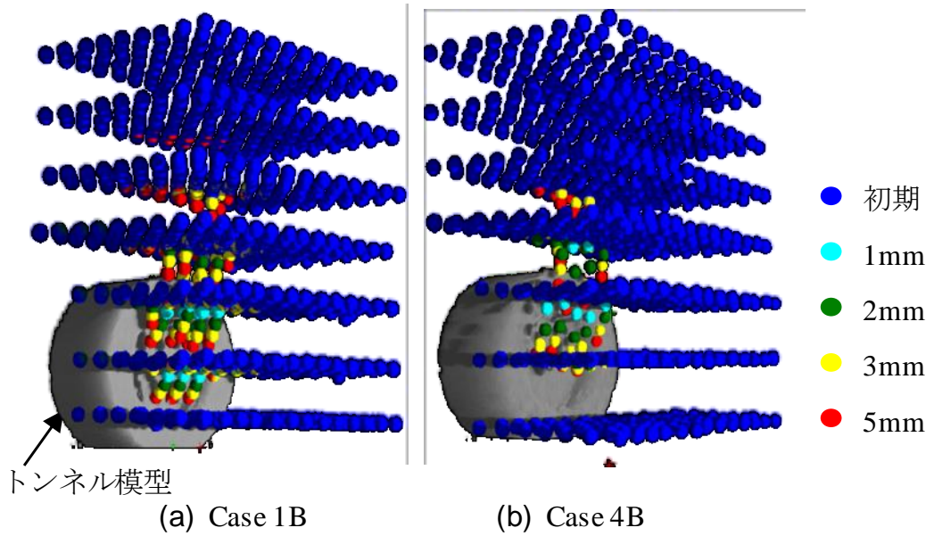
口絵写真-1 ターゲットの移動状況 8)
