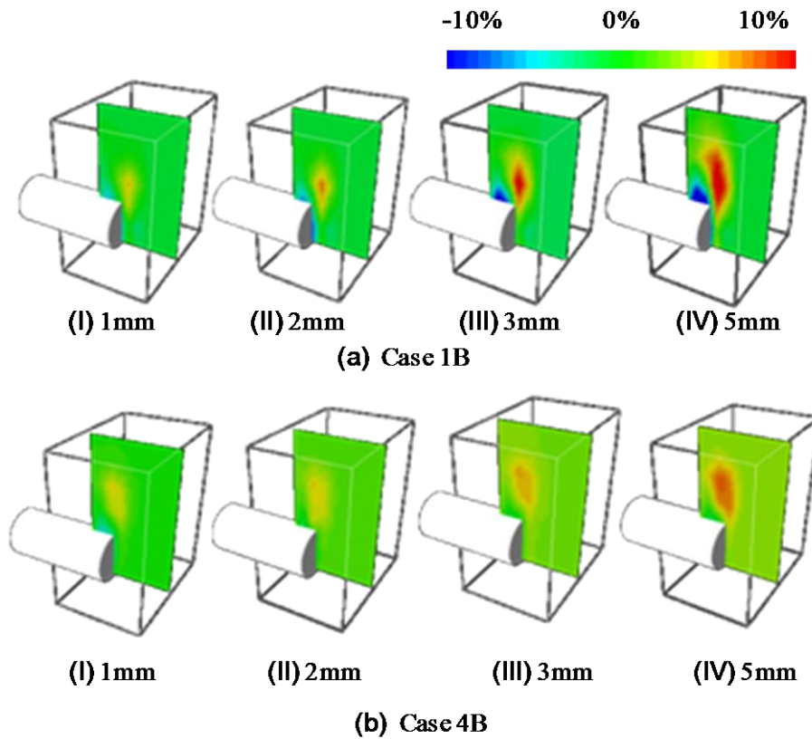
口絵写真-2 せん断ひずみ分布 8)
