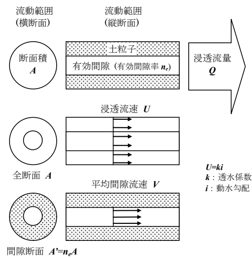
図-6.2 浸透流速と平均間隙流速の関係
