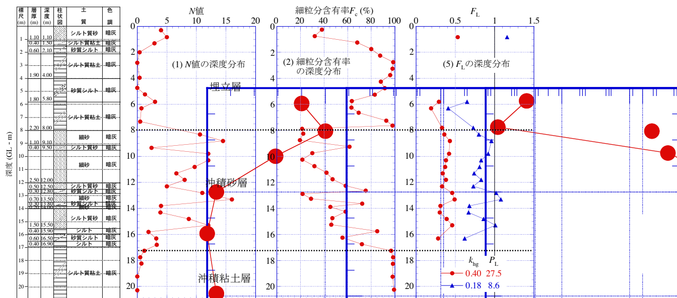
図-5 地点1の土質柱状図と N 値, F_c 値, F_L 値の深度分布
