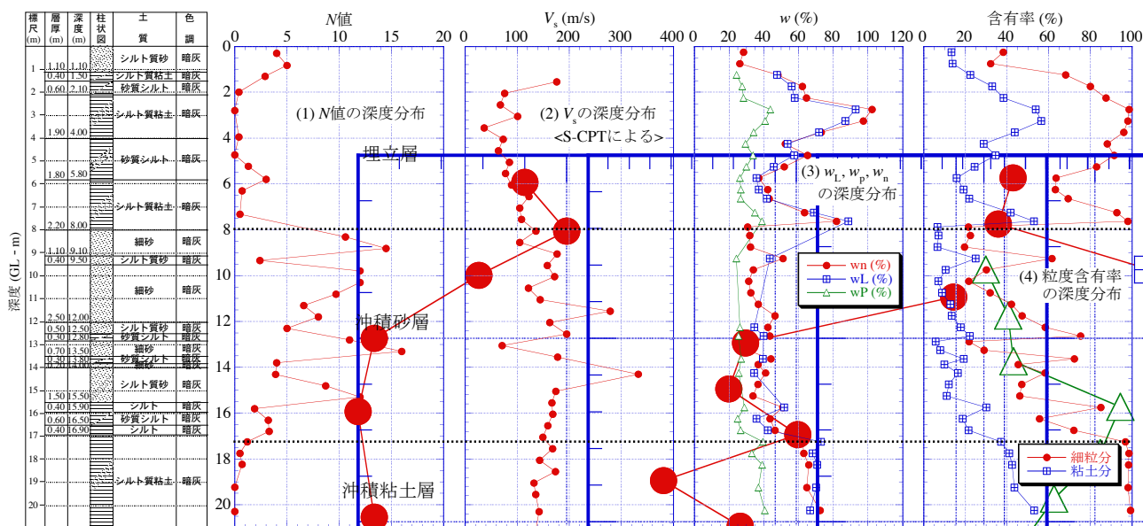
図-3 地点1の土質柱状図と N 値, V_s , 物理試験結果の深度分布
