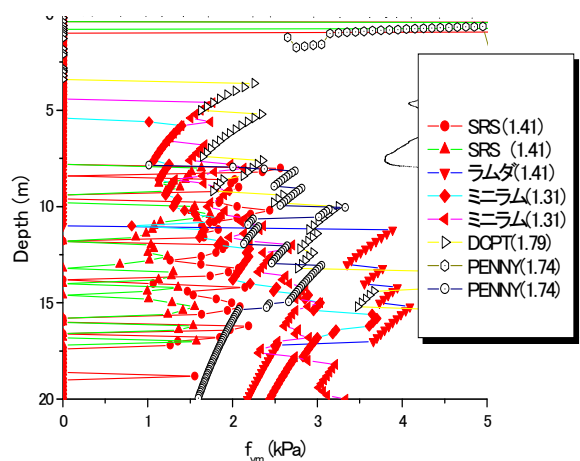
図 9 各動的貫入試験におけるロッドの摩擦 ( ) 内の数字は d/D
