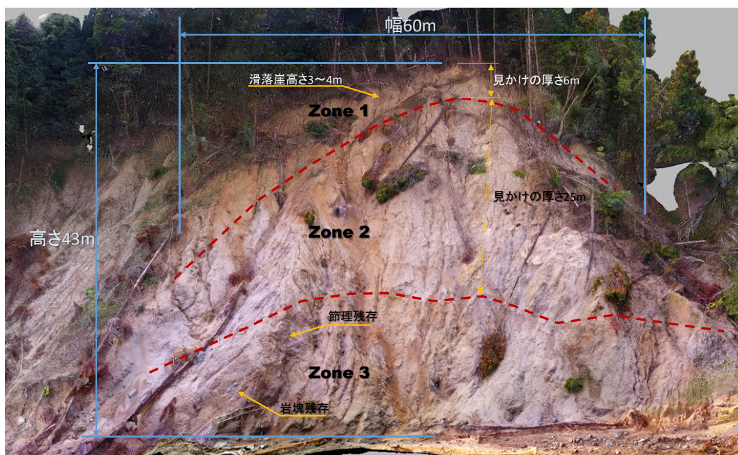
口絵写真-18 UAV簡易測量による崩壊斜面正面図と計測結果
