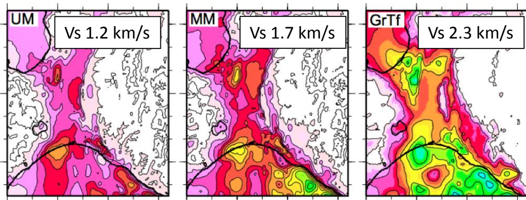
衝上断層に伴う複雑な構造
