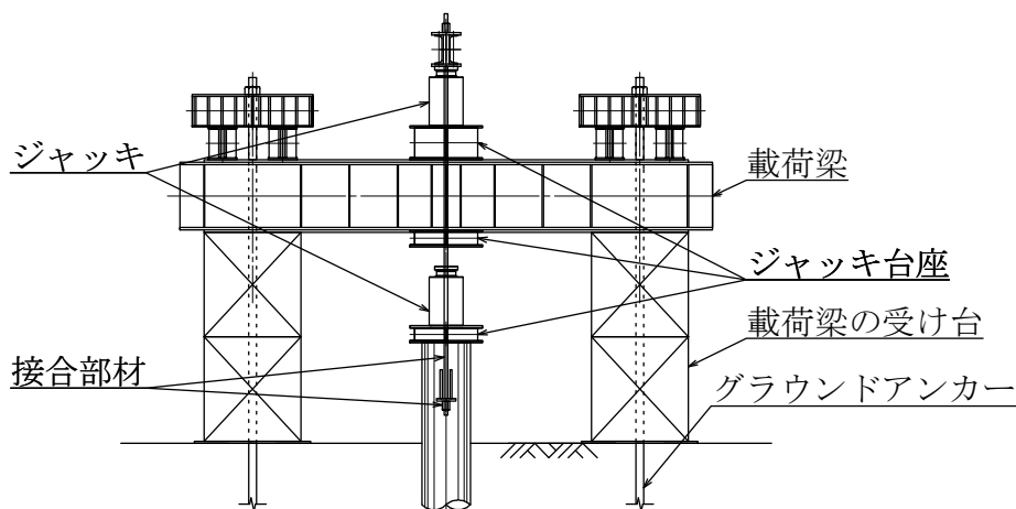
図 5—グラウンドアンカー及び反力板を用いる場合の載荷梁の支持形式の例 (押し込み側：グラウンドアンカー，引抜き側：反力板)
